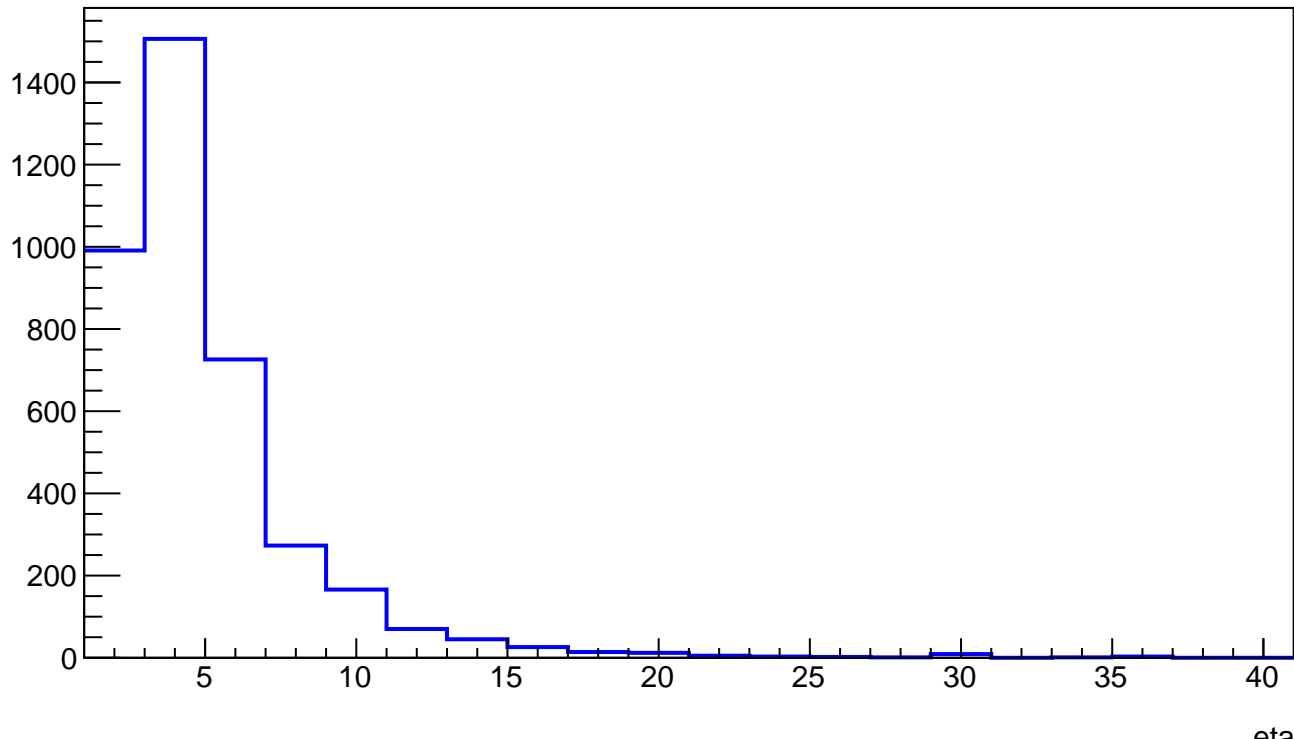
B-jet Pt second eta
