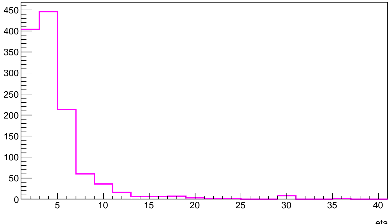
B-jet Pt third eta
