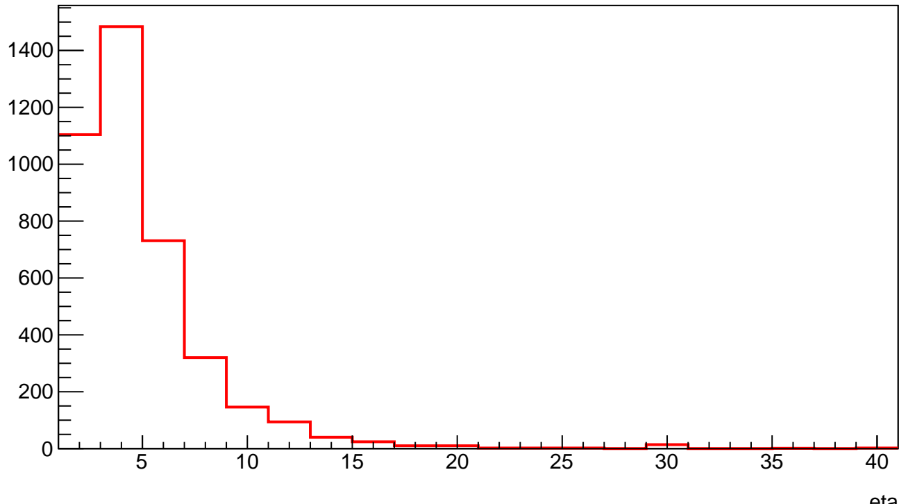
B-jet Pt first eta
