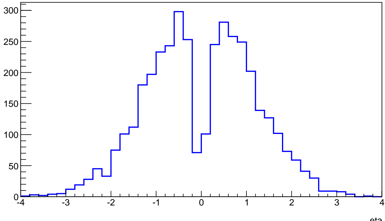
B-jet second eta
